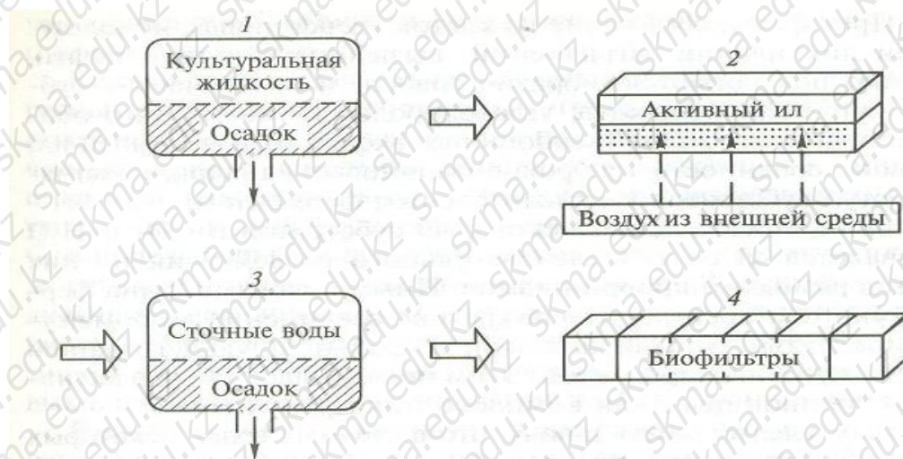
Сур. 12. Сұйық қалдықтарды биологиялық тазарту схемасы:
