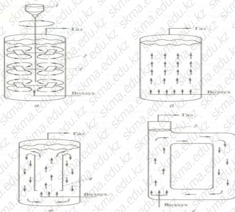
Рис. 10. Типы ферментеров (реакторов): а — реактор с механическим перемешиванием; б — барботажная колонна; в — эрлифтный реактор с внутренней рециркуляцией; г — эрлифтный реактор с внешней системой рециркуляции; 1 — пилотер; 2 — культуральная среда; 3 — насос; 4 — центральная труба; 5 — газожидкостной сепаратор; стрелками показано направление потока культуральной жидкости
