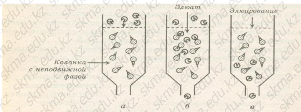
Сур. 8.3. Аффиндік хроматографияның схемалық көрінісі:
